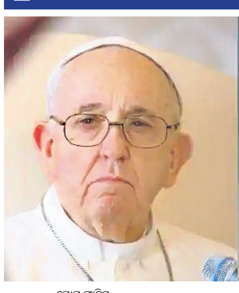
ପୋପ୍ ଫ୍ରାନ୍ସିସ୍କ
