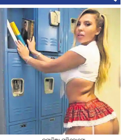
ନଟାଲିଆ ଗରିବୋଗୋ
