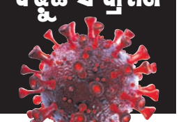
ବହୁଳ ସଂକ୍ରମଣ
