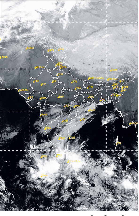
ରୁଧିର ଆପରାହ୍ନ ୫ଟାରେ ମହାକାଶରୁ ଉଦ୍ଧୋଳିତ ପାଣିପାଗର ଚିତ୍ର ।
