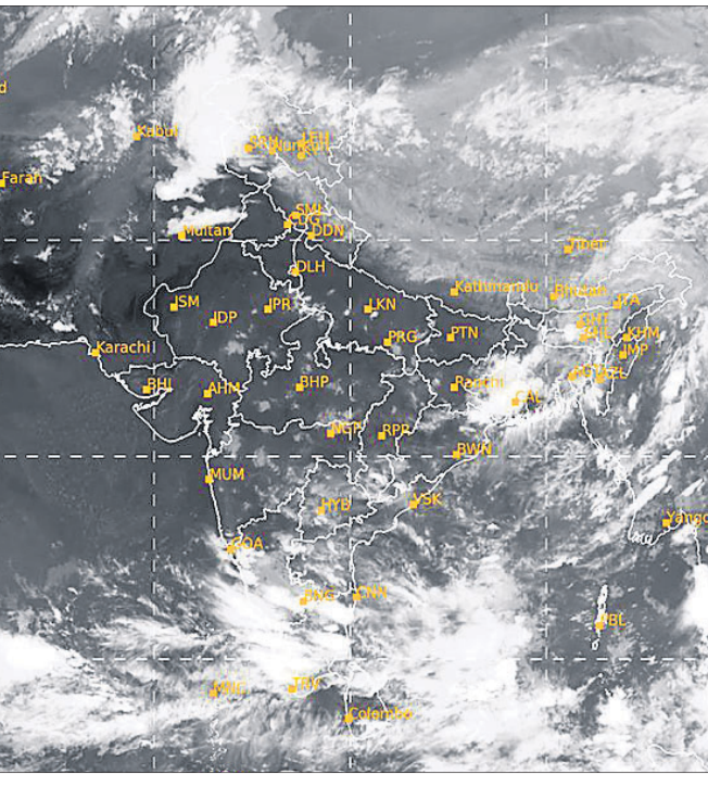
ଶନିବାର ଅପରାହ୍ଣ ୫ଟାରେ ମହାକାଶରୁ ଉତ୍ତୋଳିତ ପାଣିପାଗ ଚିତ୍ର।
