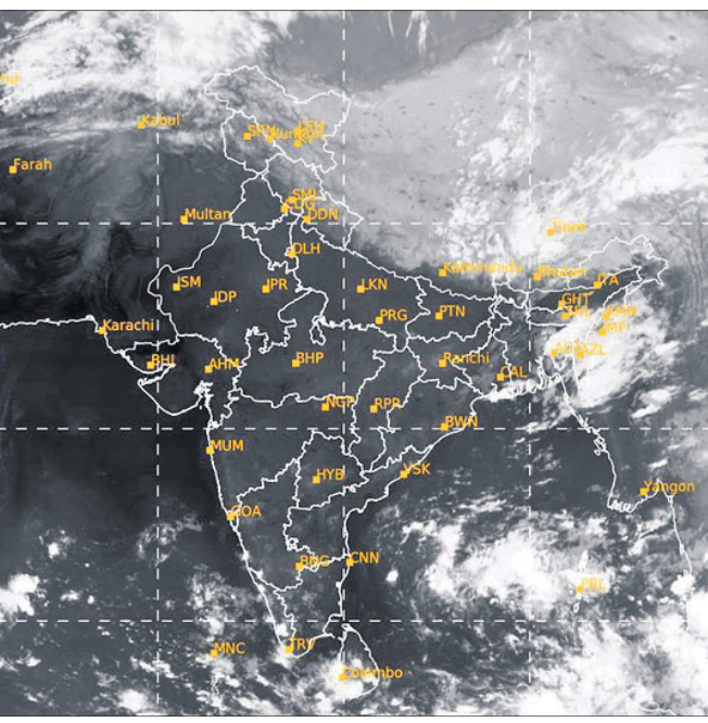
ମଙ୍ଗଳବାର ଅପରାହ୍ଣ ୫ଟାରେ ମହାକାଶରୁ ଭୌତିକ ପାଣିପାଗ ଚିତ୍ର।
