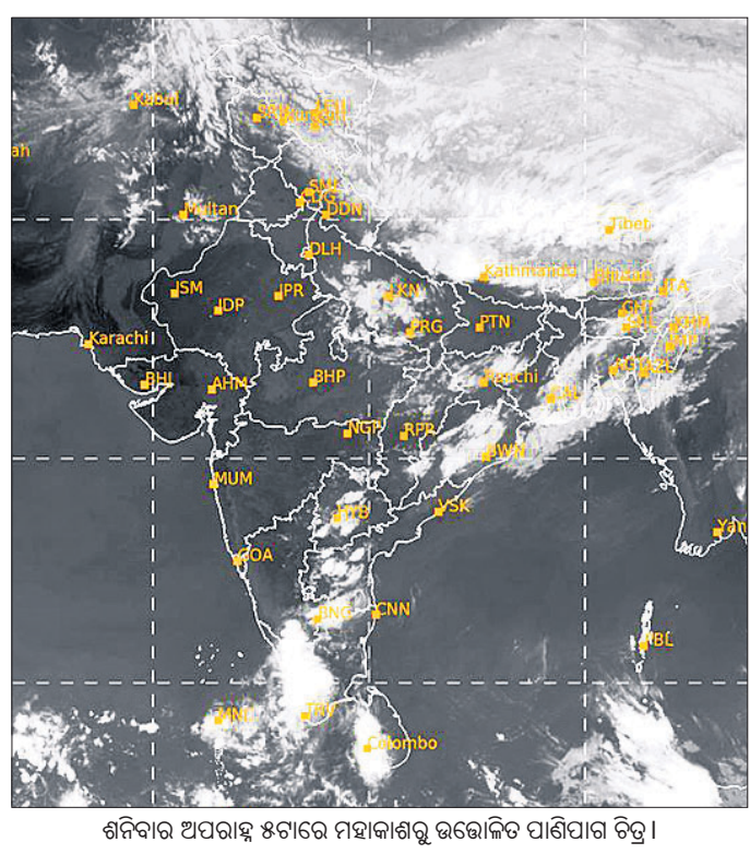
ଶନିବାର ଅପରାହ୍ଣ ୪ଟାରେ ମହାକାଶରୁ ଉତ୍ତୋଳିତ ପାଣିପାଗ ଚିତ୍ର।
