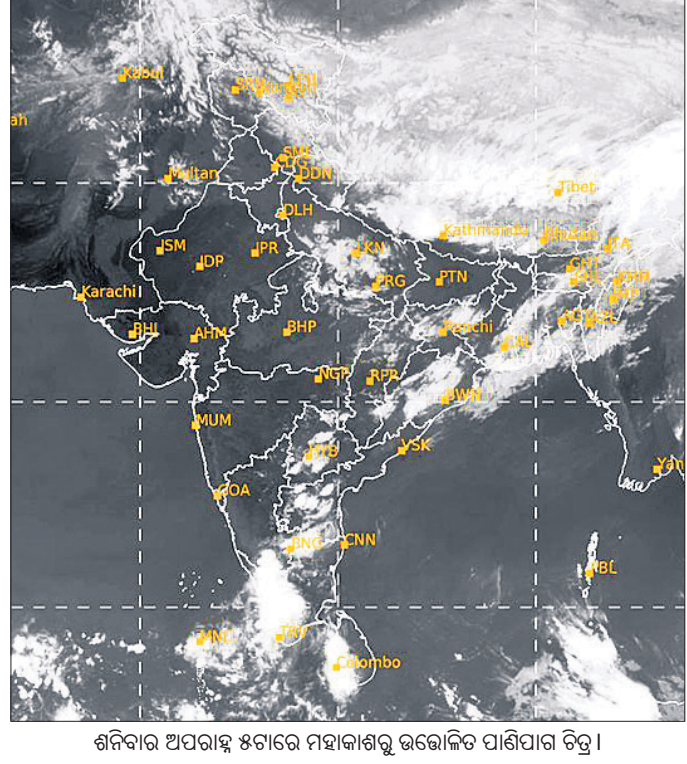
ଶନିବାର ଅପରାହ୍ନ ୫ଟାରେ ମହାକାଶରୁ ଉତ୍ତୋଳିତ ପାଣିପାଗ ଚିତ୍ର ।
