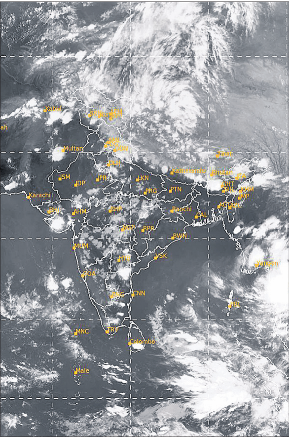
ଶୁକ୍ରବାର ଅପରାହ୍ନ ୫ଟାରେ ମହାକାଶରୁ ଉତ୍ତୋଳିତ ପାଣିପାଗର ଚିତ୍ର ।
