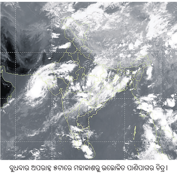
ବୁଧବାର ଅପରାହ୍ନ ୫ଟାରେ ମହାକାଶରୁ ଉଦ୍ଧୋଳିତ ପାଣିପାଗର ଚିତ୍ର ।
